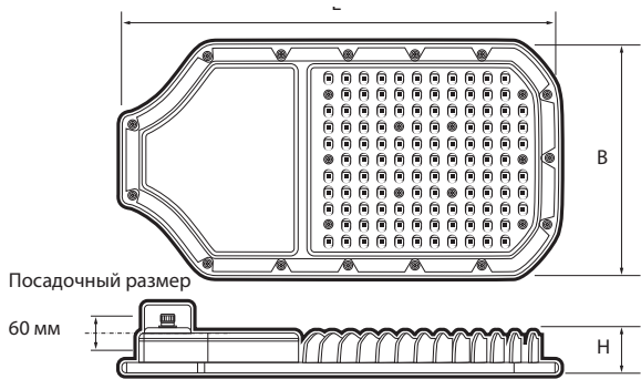
Рис.3 Размеры PSL 05-2
