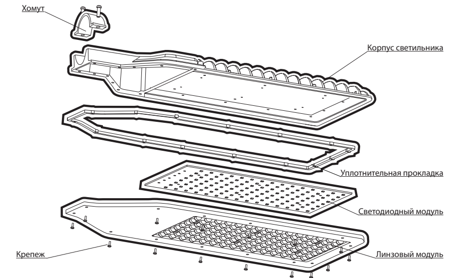
Рис.1 Взрыв-схема светильника PSL 05-2
